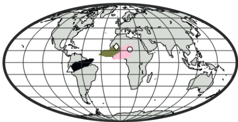
(b) MAM 2000-2015
