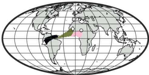
(a) DJF 2000-2015
