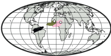
(b) MAM 2000-2015
