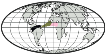
(a) DJF 2000-2015
