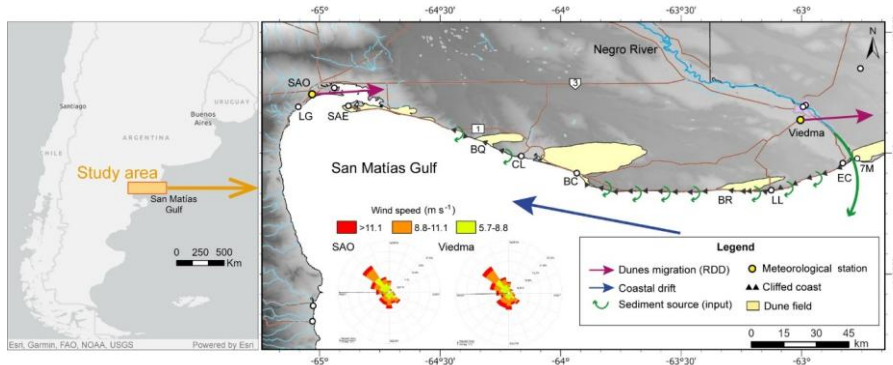
Figure 1. Study area. Meteorological stations, dunefields, and coastal villages. LG: Las Grutas, SAO: San Antonio Oeste, SAE: San Antonio Este, BQ: Bajo la Quinta, CL: Caleta de H -os Loros, BC: Bahía Creek, BR: Bahía Rosas, LL: La Lobería, EC: El Cóndor, 7M: Villa 7 de Marzo . SAO and Viedma sand roses are present. Argentina map powered by Esri. DEM basemap from Instituto Geográfico Nacional.
