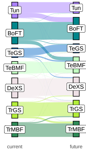
(b) RCP60
