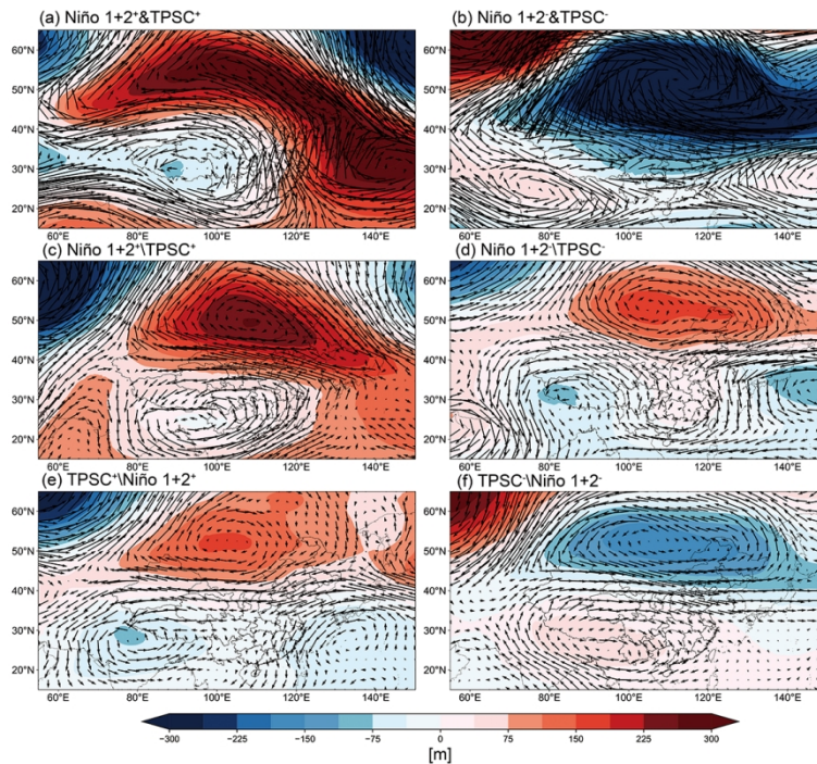
Figure 8. Composite of the geopotential height (m, shading) and wind fields ( \text{m s}^{-1} , vector) at 500 hPa for (a) Niño 1+2 + &TPSC + , (b) Niño 1+2 &TPSC - , (c) Niño 1+2 + \TPSC + , (d) Niño 1+2\TPSC - , (e) TPSC + \Niño 1+2 + , and (f) TPSC - \Niño 1+2 - .
