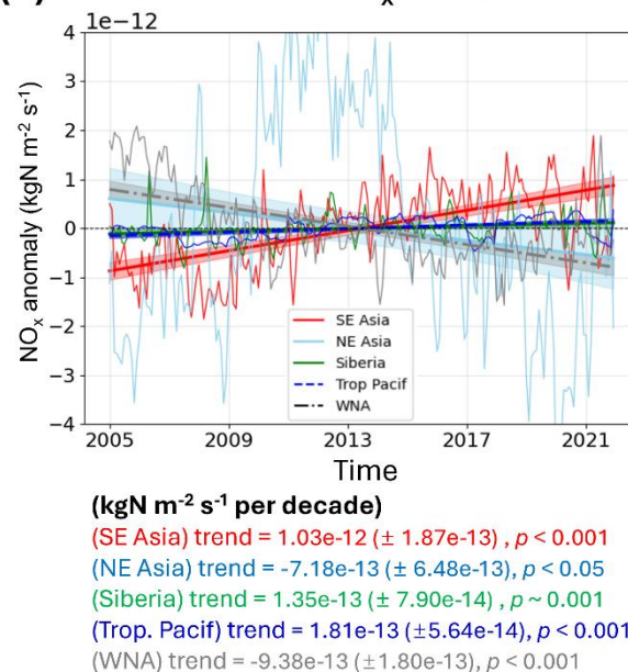
(d) TCR2 – surface NO_x emission
