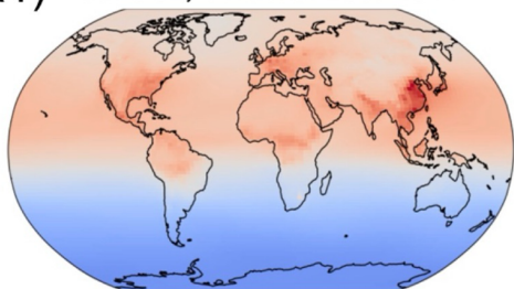
a1) atmCO 2 , CTracker 2000-2014
