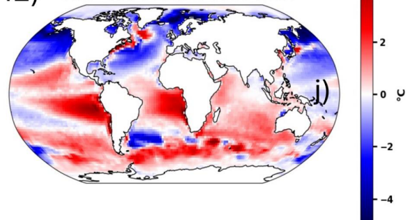
f2) eHI - WOCE2023 1991-2020
