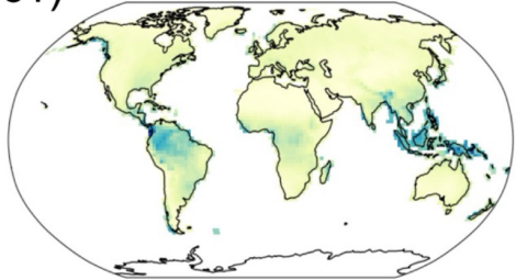
c1) Precip, GPCCv6 2001-2010
