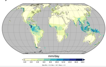
c1) Precip, GPCPv6 2001-2010
