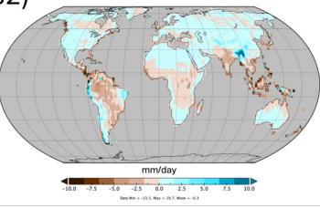
c2) eHI-Precip, 2001-2010
