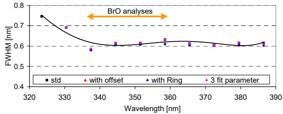
k, super-Gauss
