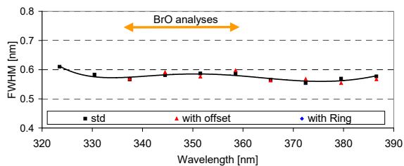
FWHM super-Gauss
