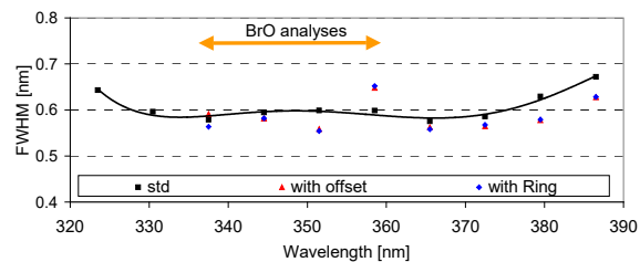
a) FWHM super-Gauss
