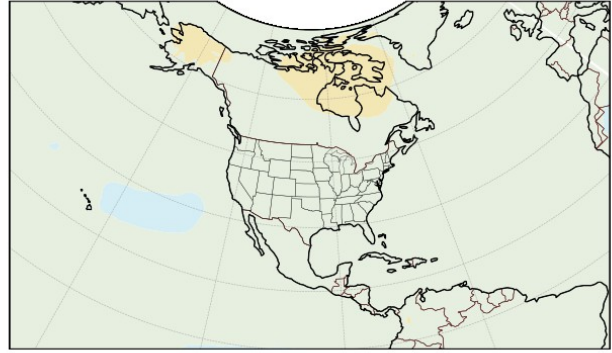
(d) WRF NoNudge - ERA-Interim, zg_{200}
