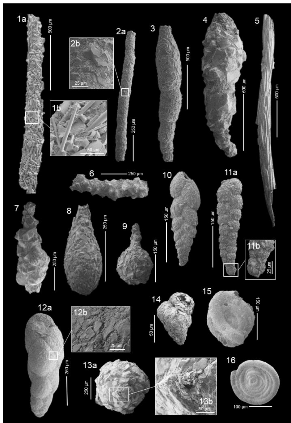
505 Plate A1. 1a-b) Rhabdammina sp. 1; 2a-b) Rhabdammina sp. 2; 3) Nodulina dentaliniformis ; 4) Reophax scorpiurus ; 5) Reophax spiculifer ; 6) Agglutinated tubular fragment; 7) Lagenammina difflugiformis ; 8) Lagenammina sp. 1; 9) Lagenammina sp. 2; 10) Pseudobolivina antarctica ; 11a-b) Spiroplectammina biformis ; 12a-b) Eggerelloides sp. 13 a-b) Psammospheara fusca ; 14) Rhumlerella sp.; 15) Ammovertillina sp.; 16) Ammodiscus incertus .
