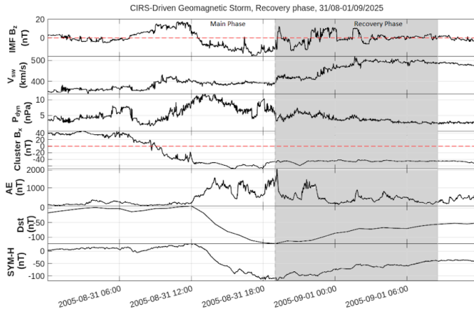
Cluster orbit 2005 242 (08/30) 11:00 UT to 2005 244 (09/01) 20:05 UT
