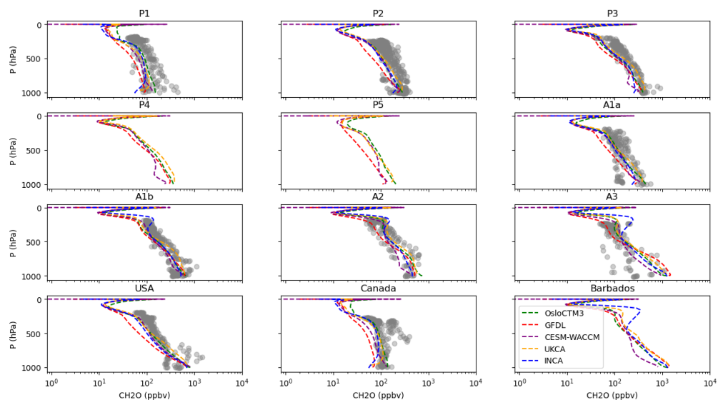
ATom4 (spring)
