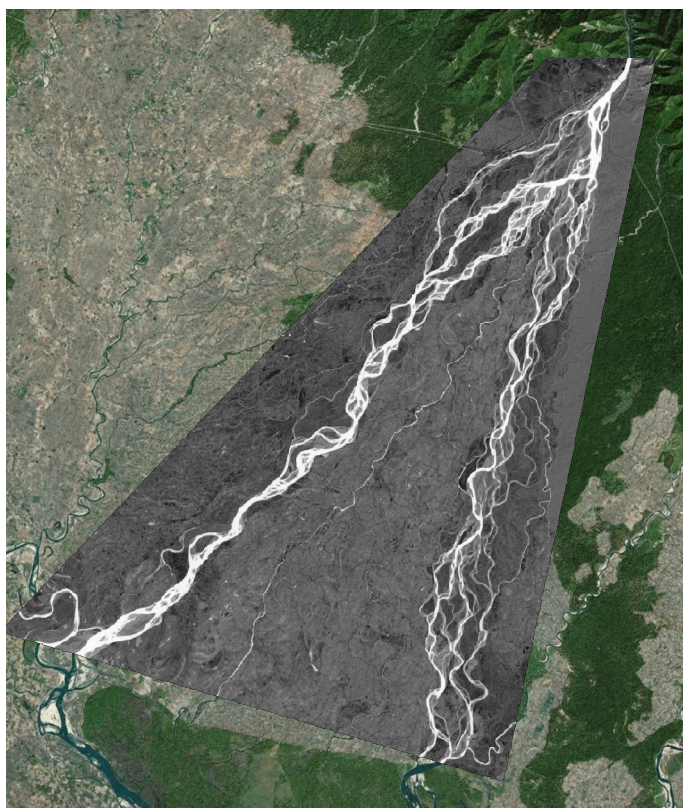
Landsat 8 2018-10-04 (AWEI)
