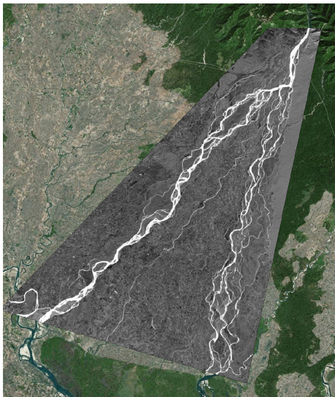
Landsat-8 2016-10-30 (AWEI)
