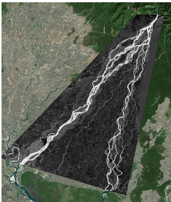
Landsat-8 2021-10-28 (AWEI)
