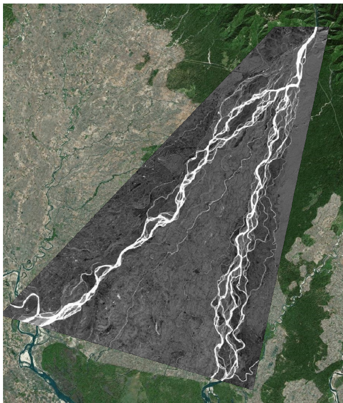
Landsat 8 2014-10-09 (AWEI)
