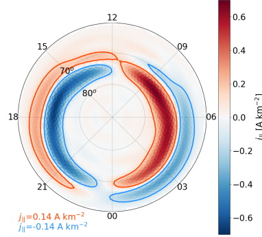
(d) AMPS field-aligned current density
