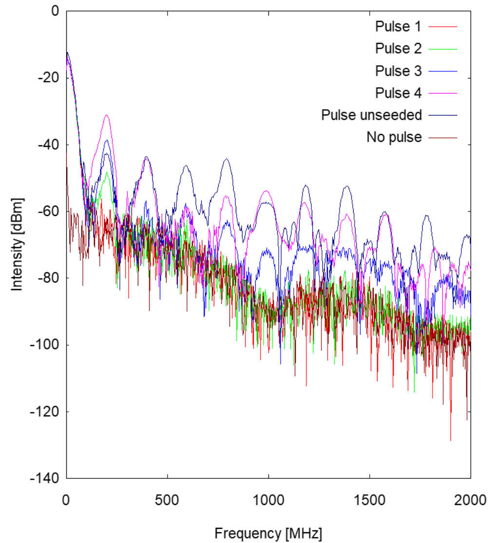
Spectra
