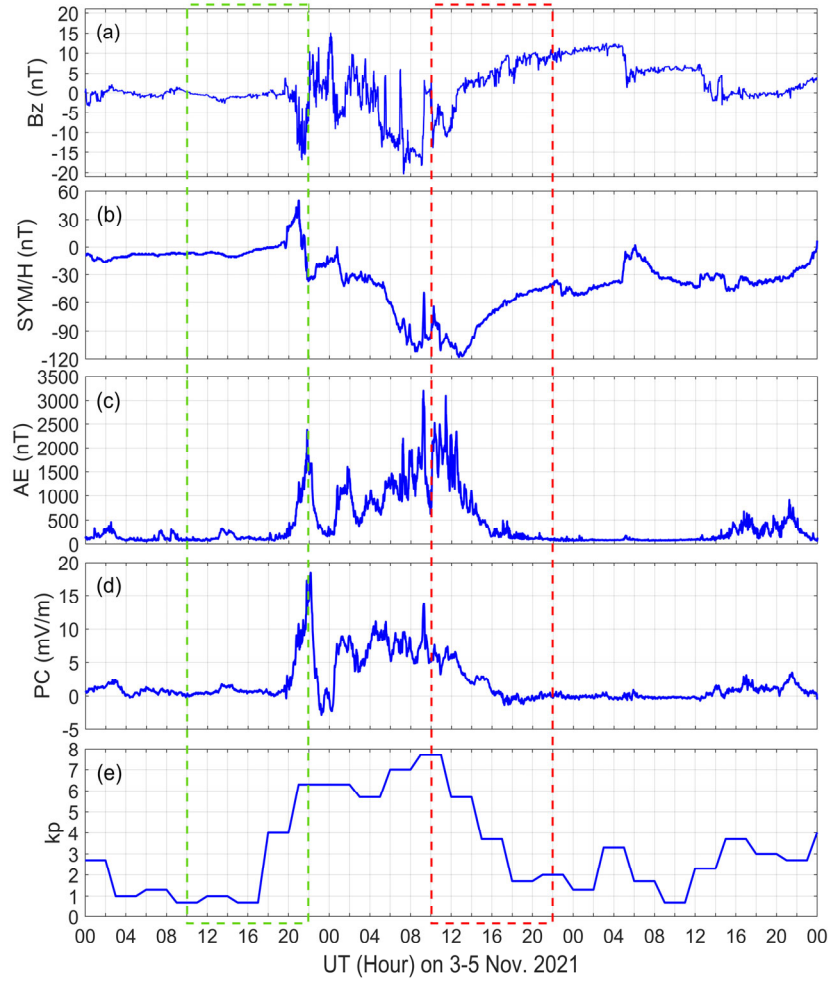
Figure 1. Geomagnetic indexes. (a) Bz, (b) SYM/H, (c) AE, (d) PC and (e) kp indexes on 3-5 November 2021.
