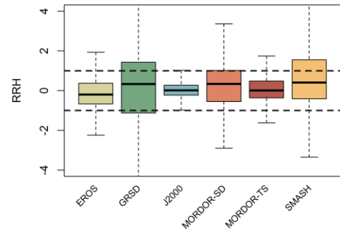
(d) q_a CDF-t
