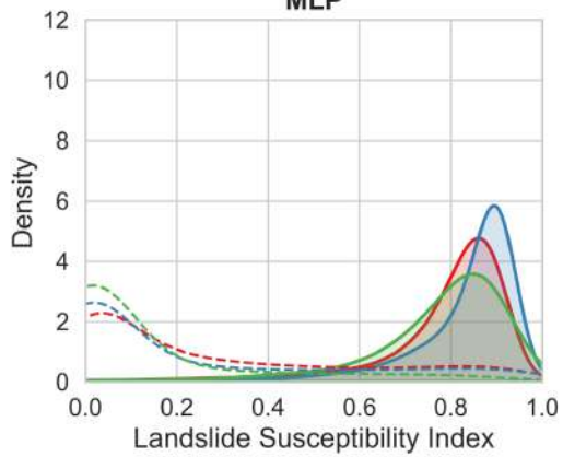
MLP
