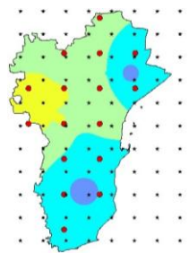
d. Tuticorin - MSWEP
