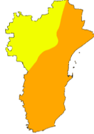
h. Tuticorin – NCEP2
