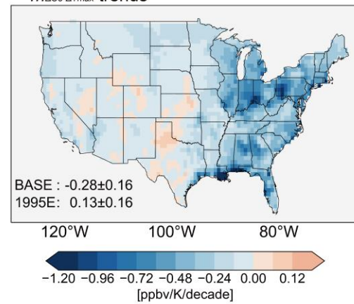
(d) Contribution of NO x emission reduction to m_{\Delta O_3-\Delta T_{max}} trends
