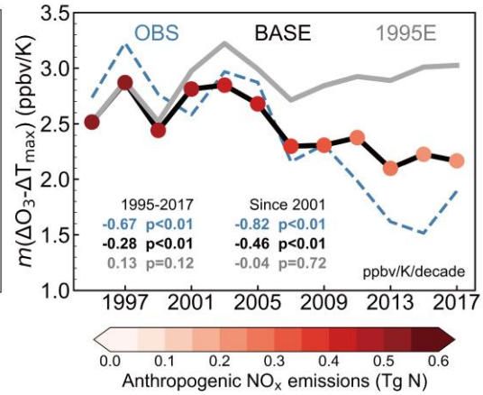
(d) Contribution of NO x emission reduction to m_{\Delta O_3-\Delta T_{max}} trends
