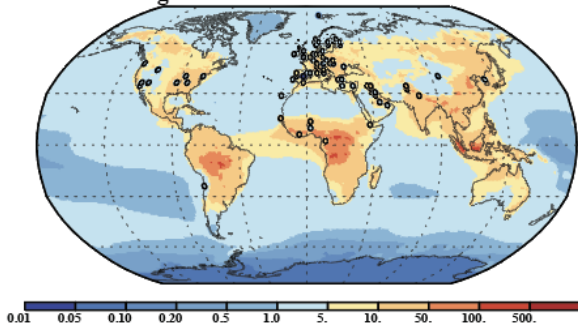
g. Na PM10 \mu\text{g}/\text{m}^3
