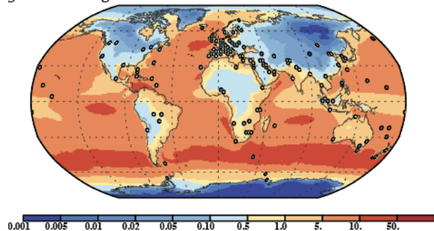
g. Na PM10 \mu\text{g}/\text{m}^3
