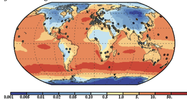
g. Na PM10 \mu\text{g}/\text{m}^3
