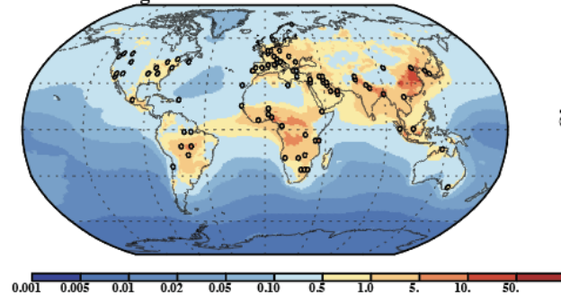
e. OM PM10 \mu\text{g}/\text{m}^3
