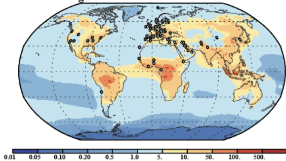
g. Na PM10 \mu\text{g}/\text{m}^3
