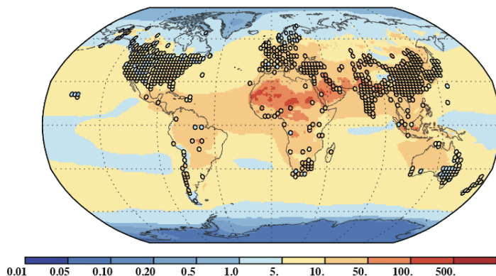
b. PM 2.5 (ug/m 3 )
