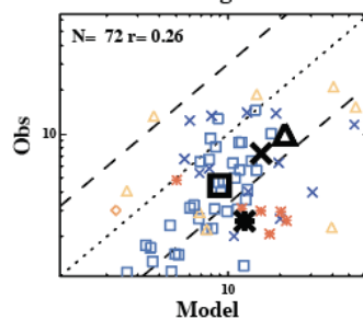
f. OM PM10 \mu\text{g}/\text{m}^3
