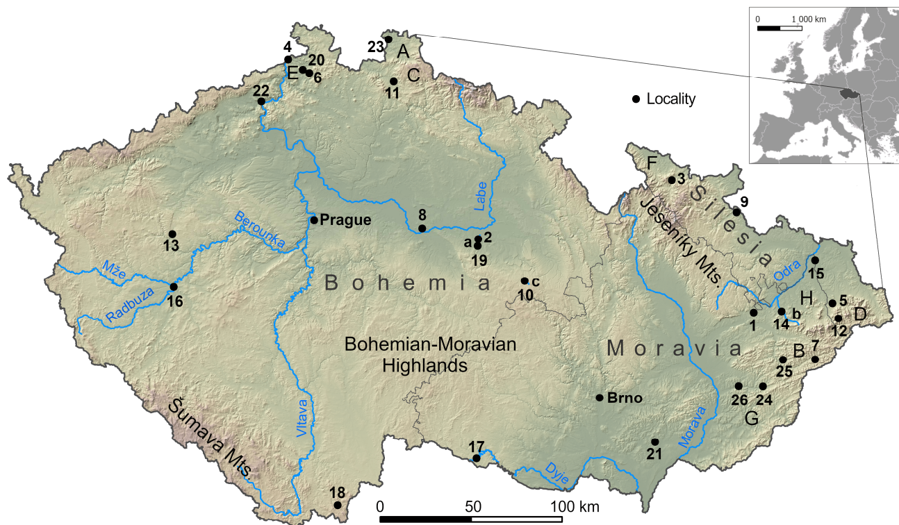
Figure 1: Location of places, watercourses and geomorphological units in the Czech Republic mentioned in the text. Localities: 1 – Běloutín, 2 – Čepí, 3 – Česká Ves, 4 – Hřensko, 5 – Janovice, 6 – Janská, 7 – Karolinka, 8 – Konárovice, 9 – Krnov, 10 – Krouna (Rychnov), 11 – Liberec, 12 – Lysá hora, 13 – Mladotice, 14 – Nový Jičín, 15 – Ostrava, 16 – Plzeň, 17 – Podhradí nad Dyjí, 18 – Pohorská Ves, 19 – Rozhovice, 20 – Srbská Kamenice, 21 – Šardice, 22 – Ústí nad Labem, 23 – Višňová, 24 – Vizovice, 25 – Vsetín, 26 – Zlín. Watercourses: a – Dubanka, b – Jičínka, c – Rychnovský potok. Geomorphological units: A – Frýdlantská pahorkatina Hilly Land, B – Hostýnsko-Vsetínská hornatina Mts., C – Jizerské hory Mts., D – Moravian-Silesian Beskids, E – Labské pískovce Sandstones, F – Rychlebské hory Mts., G – Vizovická vrchovina Highlands, H – Západobeskydské podhůří Foothills.
