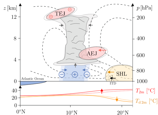
(a) Deep-cloud parameters ( entrorg, zvz0i )
