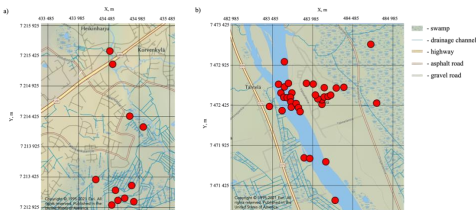
210 Figure 7: Locations of the frost quakes, detected on 6.1. 2023: a) Talvikangas; b) Tähtelä.
