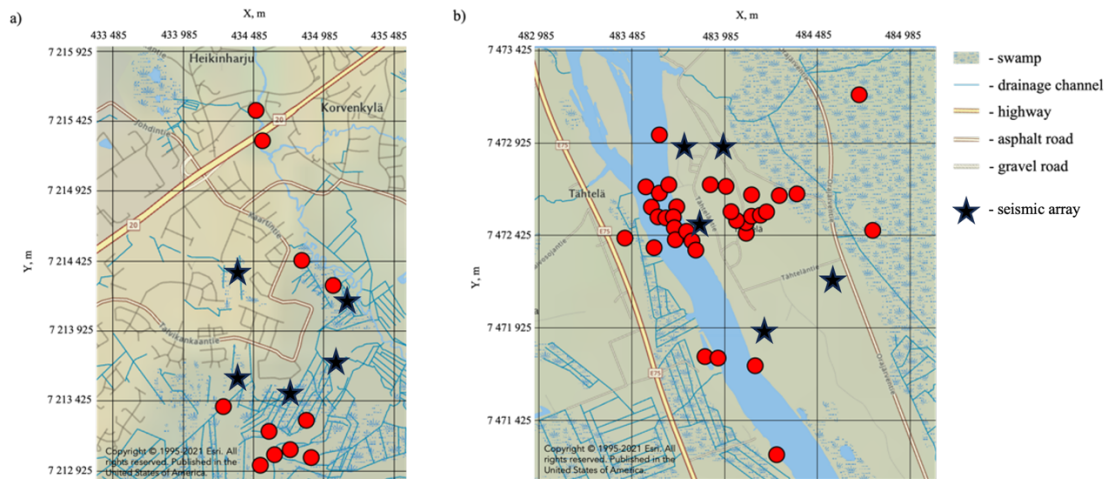
220 Figure 7: Locations of the frost quakes, detected on 6.1. 2023: a) Talvikangas; b) Tähtelä.
