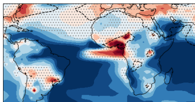
(d) GISS O 3
