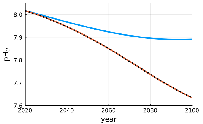
(d) Upper ocean layer pH
