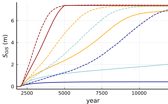
(d) Greenland ice sheet contribution to sea level rise
